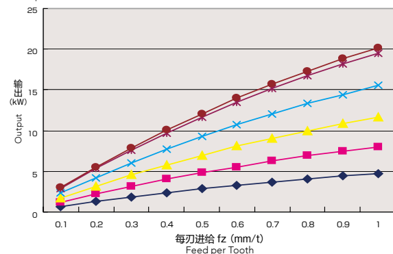
FC250 机械主轴用电机 (输出) 表
