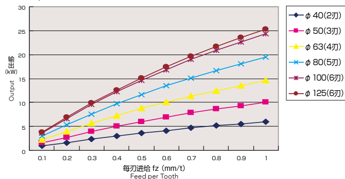
S50C 机械主轴用电机 (输出) 表
