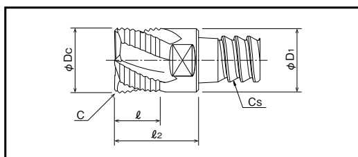
PXNL 不等导程 4刃 小螺旋角 粗加工型 Variable Lead, Four Flutes, Low Helix, Roughing Type
