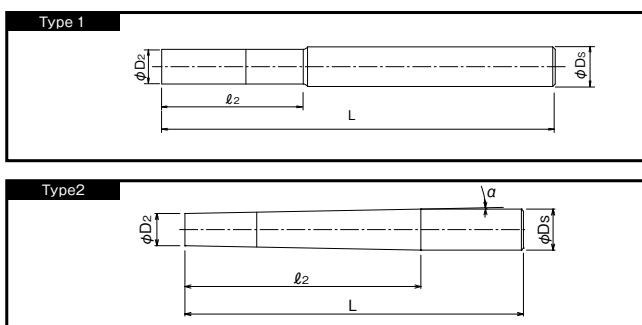
■形状尺寸表 Specification
